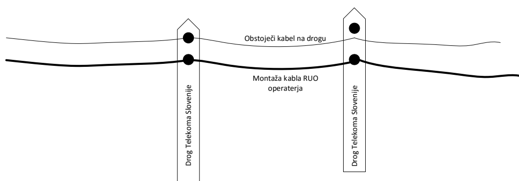
Slika 29: Pravilni prehod kabla na drogu
