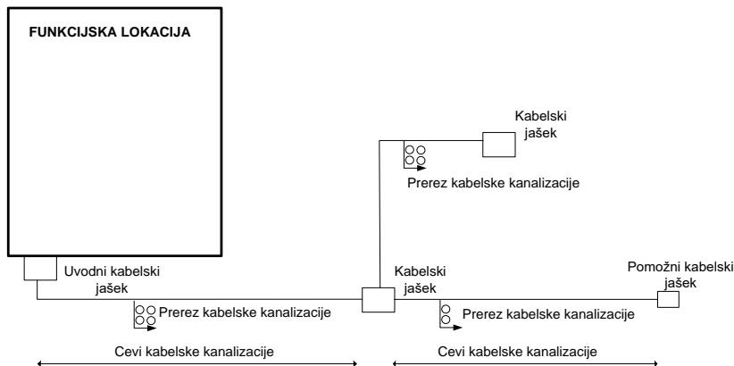
Slika 7: Kabelska kanalizacija
