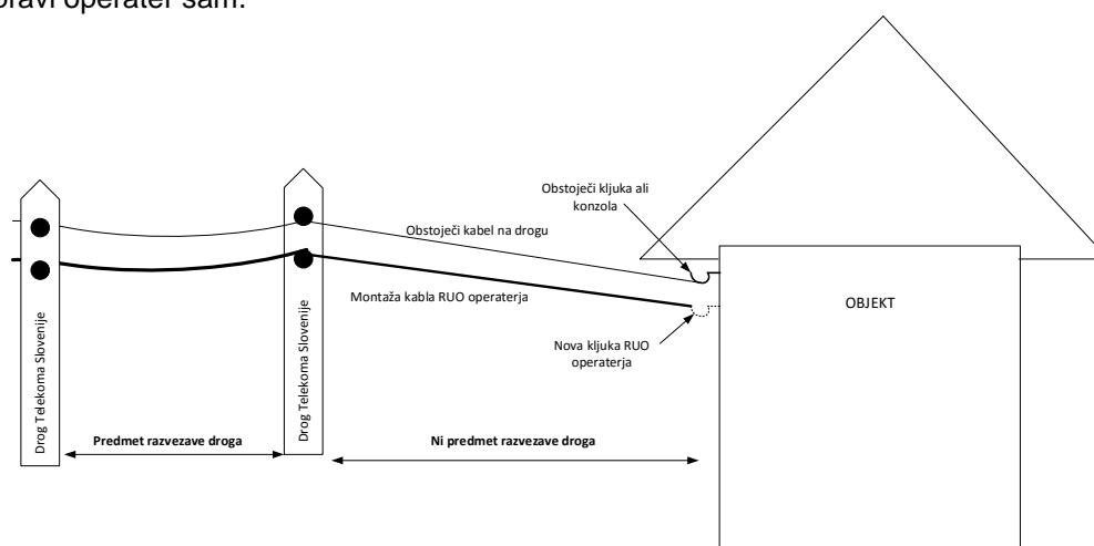
Slika 27: Razmejitvena točka med drogom in objektom
