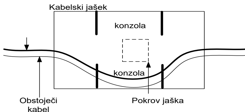
Slika 25: Pravilni prehod skozi jašek
