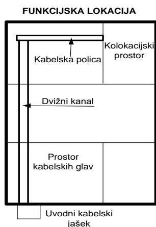
Slika 8: Povezava znotraj funkcijske lokacije
