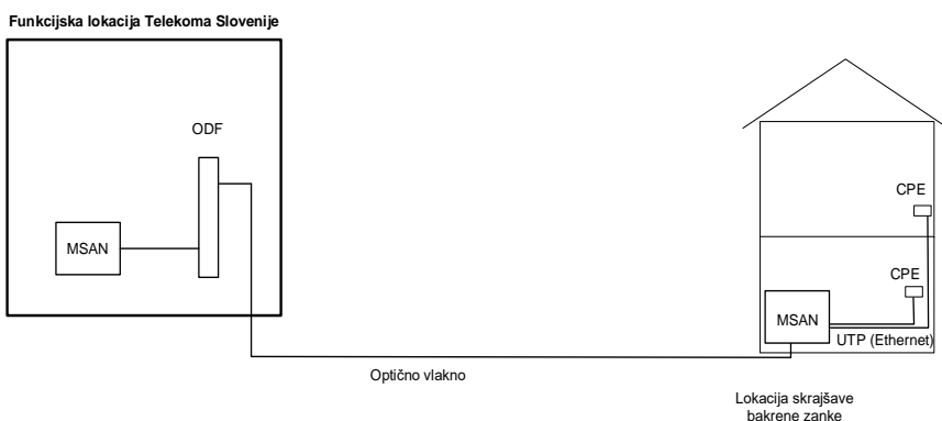
Slika 3: Topologija skrajšave zanke v dostopnem bakrenem kabelskem omrežju – tip FTTF
