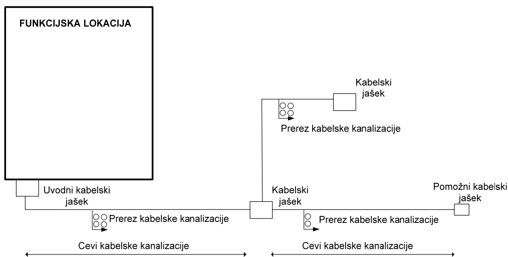
Slika 3: Kableska kanalizacija
