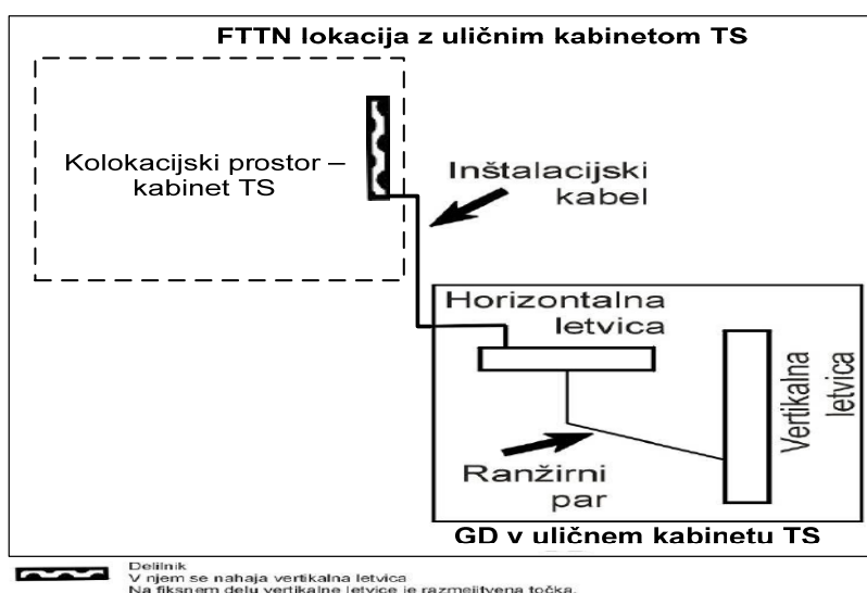
Slika 16: FTTN skupna lokacija (prostor v uličnem kabinetu) tipa E
