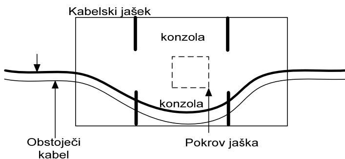
Slika 20: Pravilni prehod skozi jašek
