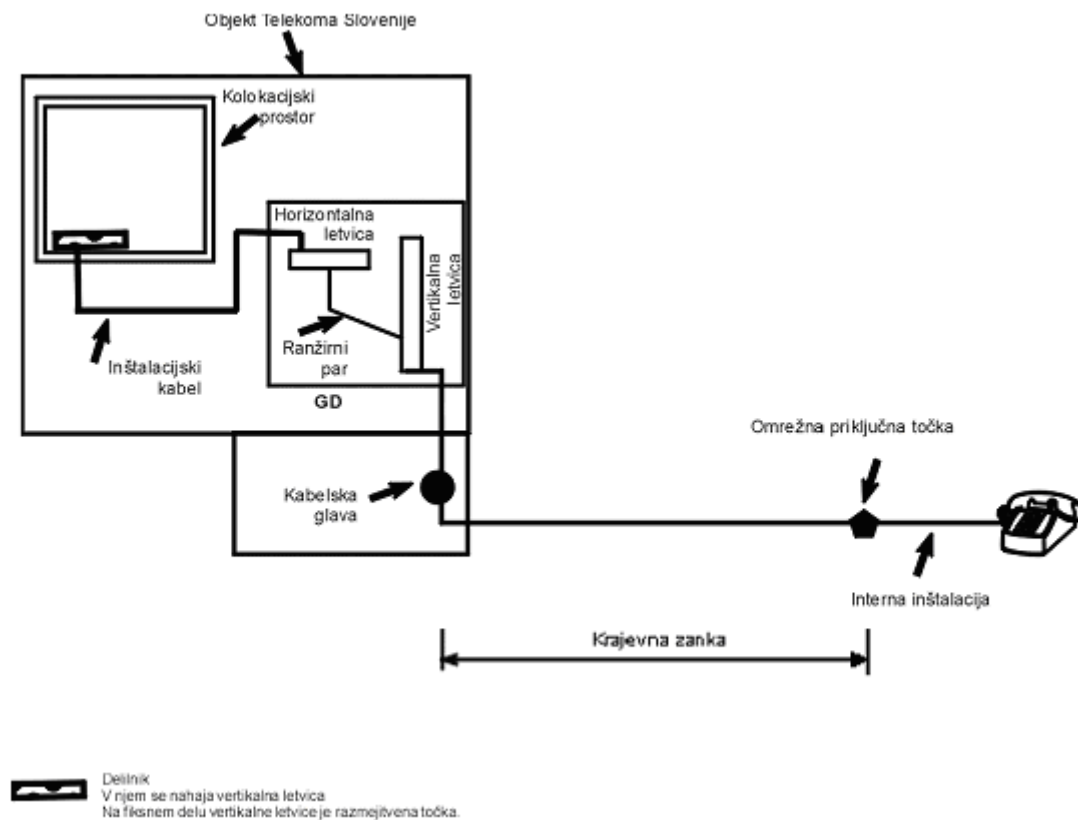
Slika 2: Topologija dostopovnega omrežja Telekom Slovenije (za primer povsem razvezanega dostopa)
