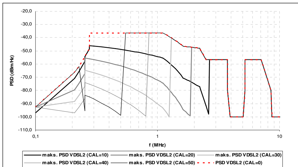
Graf PSD maske (DS) za različne vrednosti slabljenja CAL
