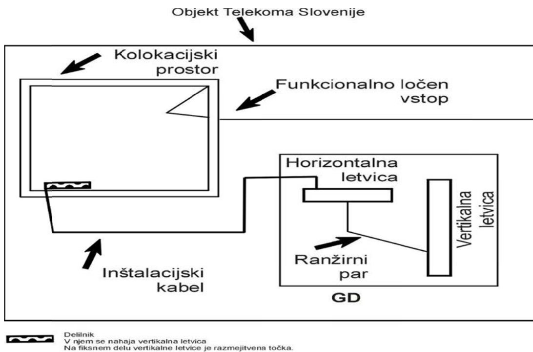
Slika 11: Prostor skupne lokacije tipa A
