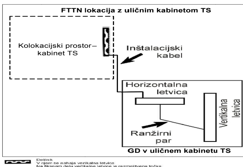
Slika 16: FTTN skupna lokacija (prostor v uličnem kabinetu) tipa E
