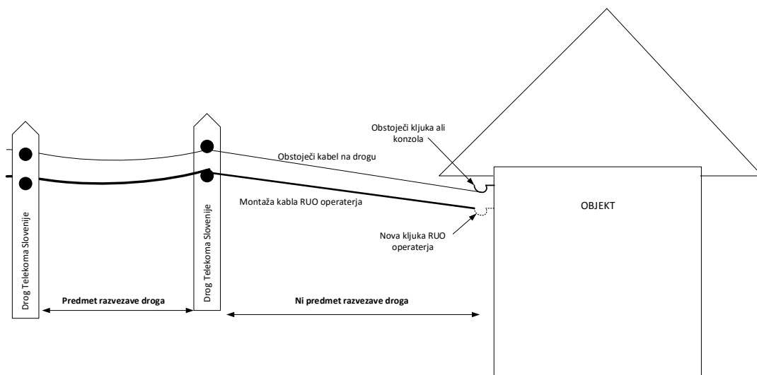
Slika 27: Razmejitvena točka med drogom in objektom
