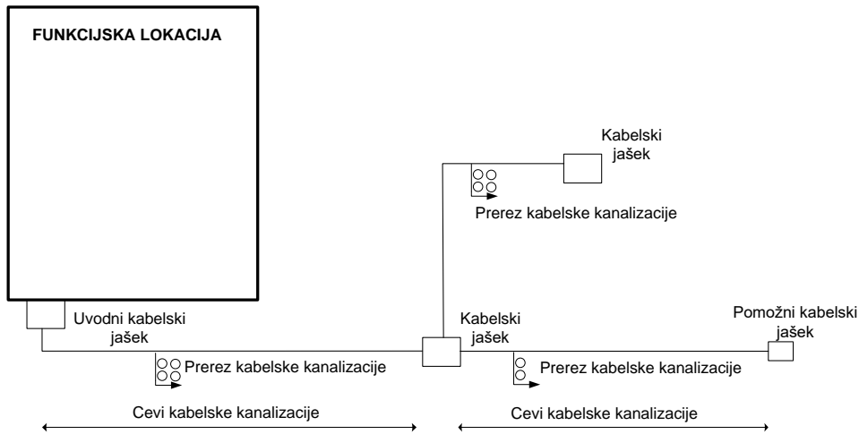
Slika 7: Kabelska kanalizacija
