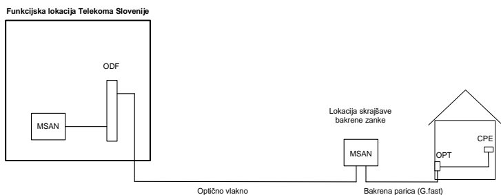
Slika 2: Topologija skrajšave zanke v dostopnem bakrenem kabelskem omrežju – tip FTTC
