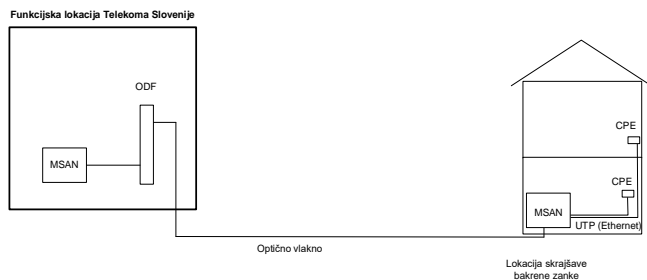
Slika 3: Topologija skrajšave zanke v dostopnem bakrenem kabelskem omrežju – tip FTTF
