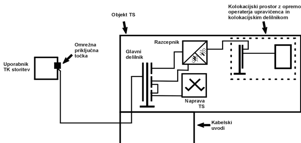
Slika 11: Sodostop do bakrene krajevne zanke
