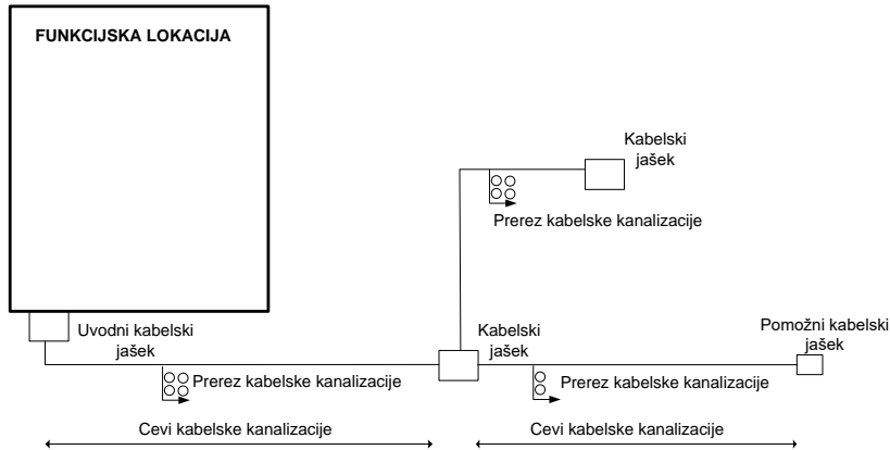
Slika 7: Kableska kanalizacija
