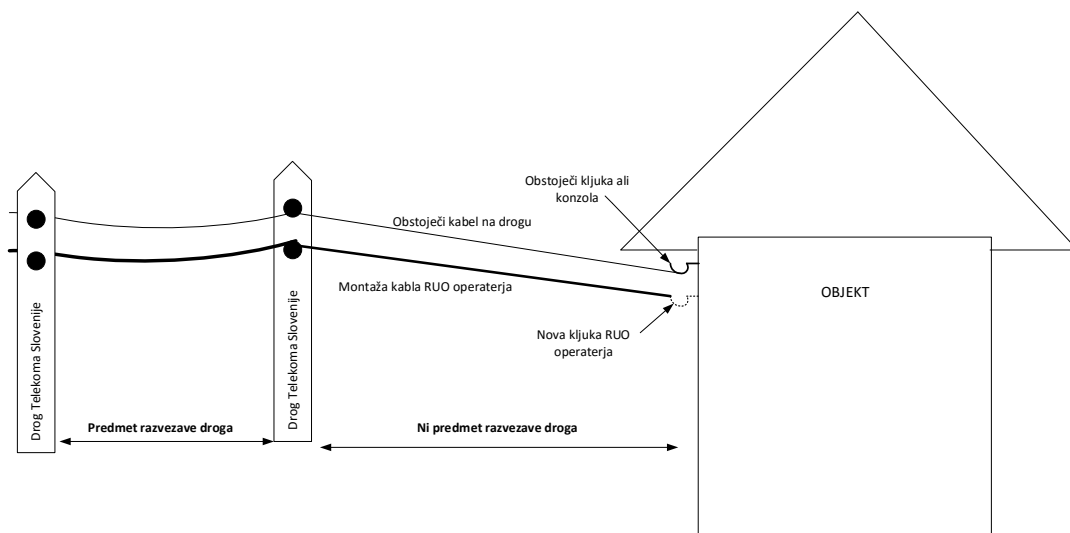
Slika 27: Razmejivna točka med drogom in objektom
