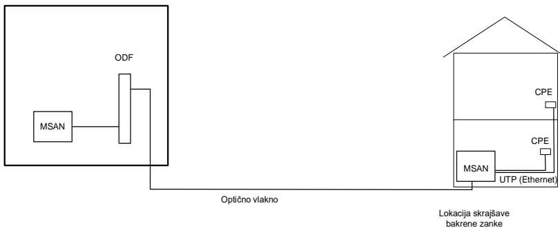
Slika 3: Topologija skrajšave zanke v dostopnem bakrenem kabelskem omrežju – tip FTTPdp
