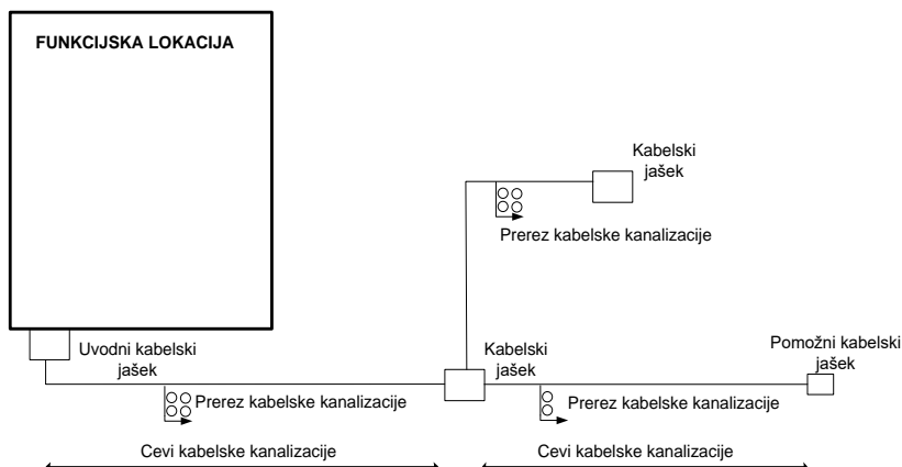
Slika 7: Kabelska kanalizacija
