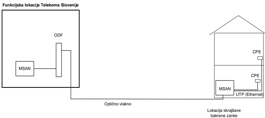
Slika 3: Topologija skrajšave zanke v dostopnem bakrenem kabelskem omrežju – tip FTTP
