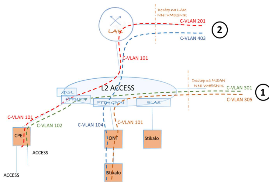
Slika 1: Zagotavljanje logične povezave (1 – dostop do aktivnega dostopnega vozlišča, 2 – dostop do robnega vozlišča)
