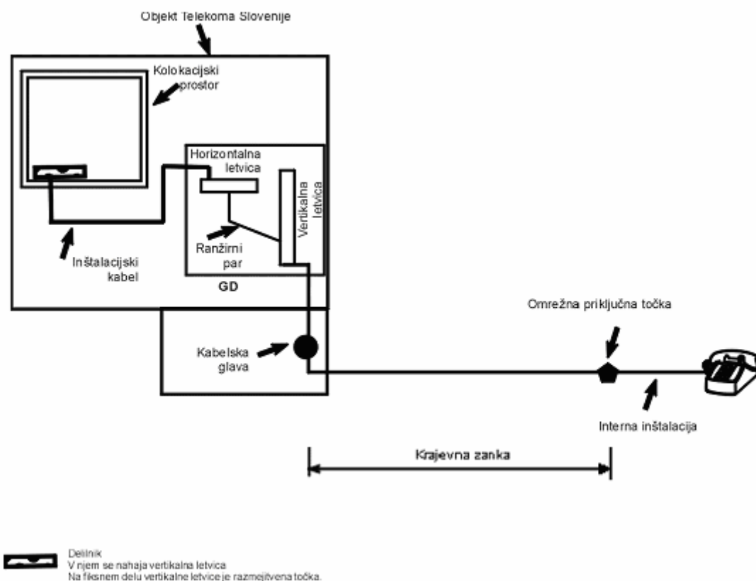
Slika 2: Topologija dostopnega omrežja Telekom Slovenije (za primer polnega dostopa)
