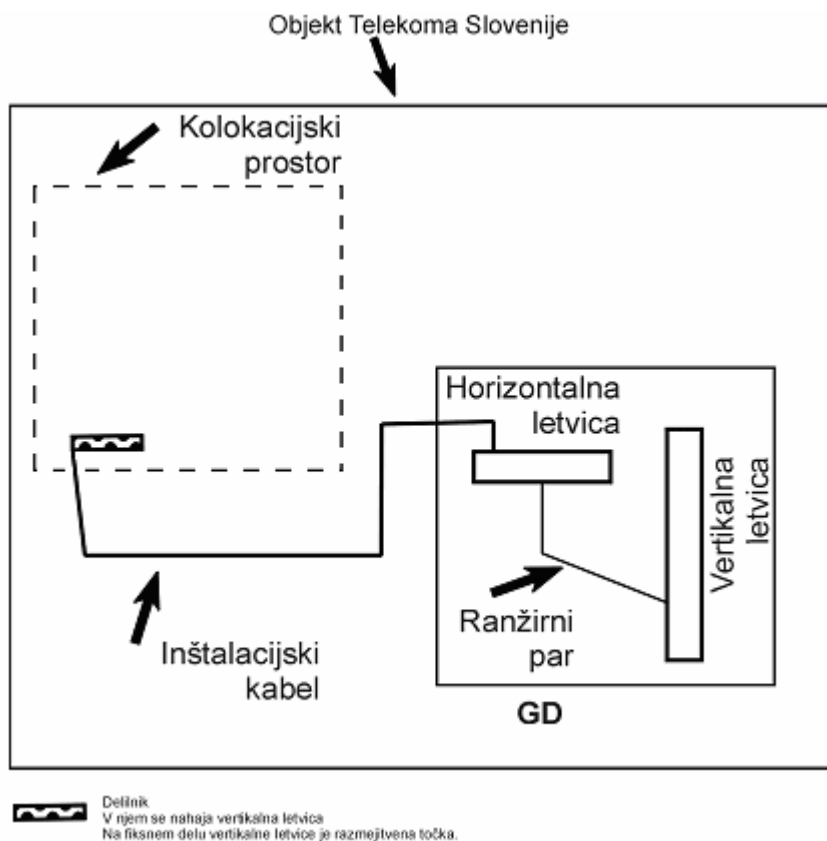
Slika 5c: Kolokacijski prostor tipa C
