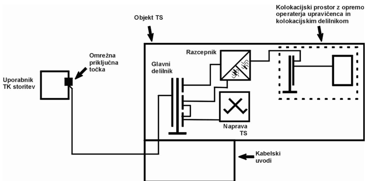
Slika 4: Skupi razvezani dostop
