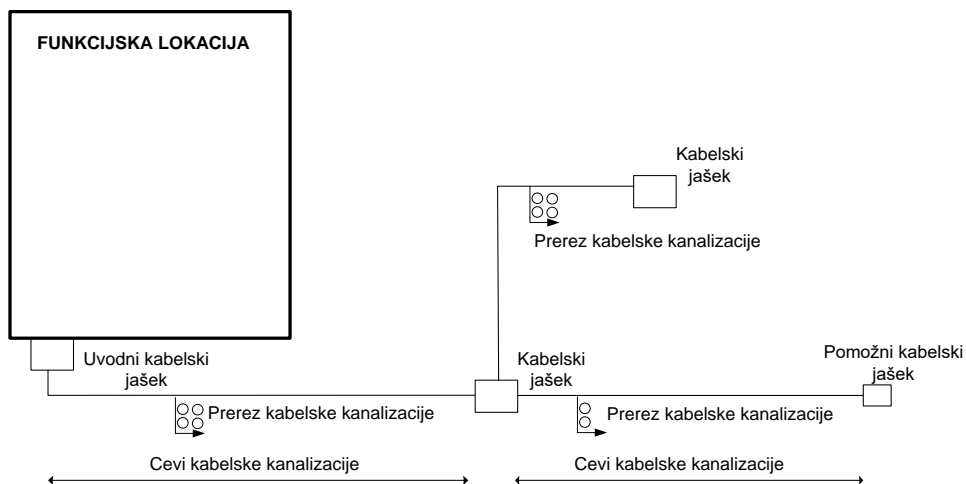
Slika 7: Kableska kanalizacija
