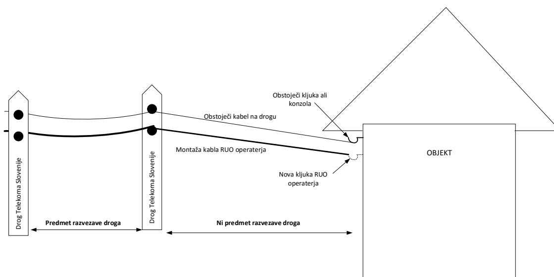
Slika 26: Razmejitvena točka med drogom in objektom
