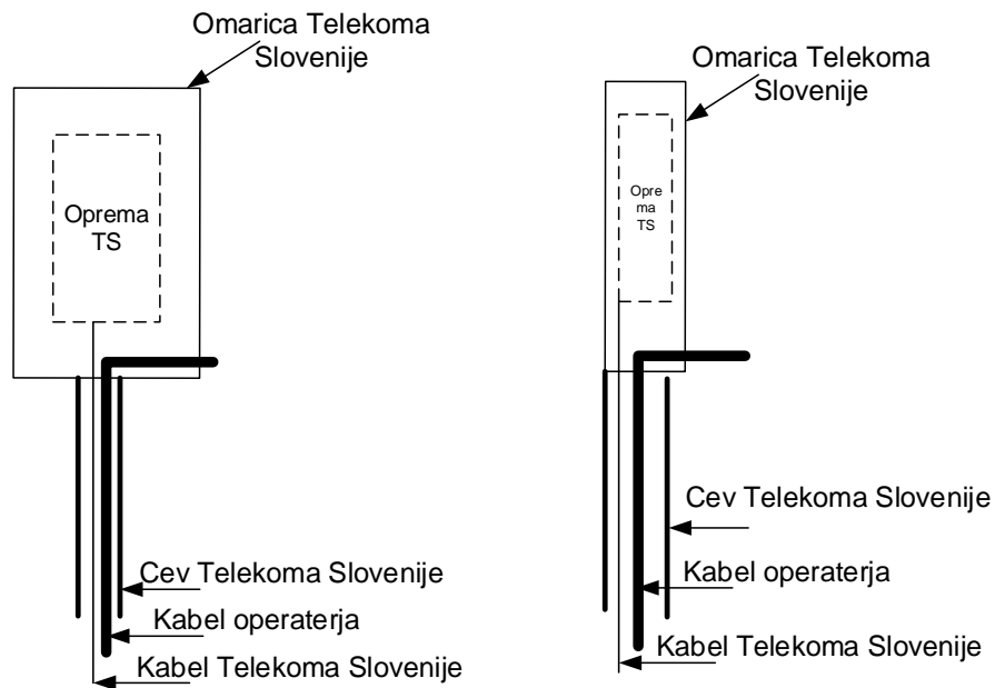
Slika 21: Prikaz dovoljenega prehoda kabla operaterja skozi omarico Telekom Slovenije – prednji pogled in stranski pogled
