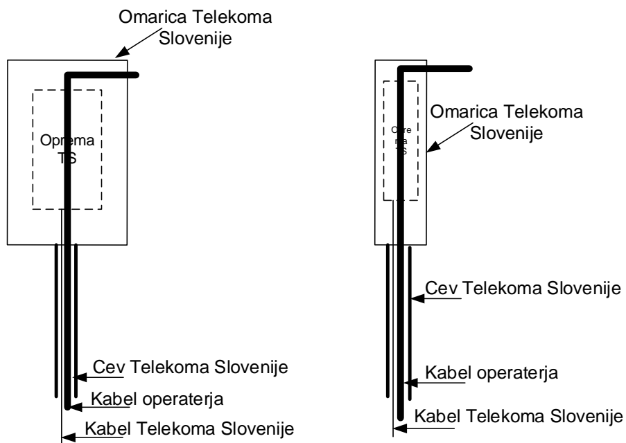
Slika 22: Prikaz nedovoljenega prehoda kabla operaterja skozi omarico Telekom Slovenije – prednji pogled in stranski pogled
