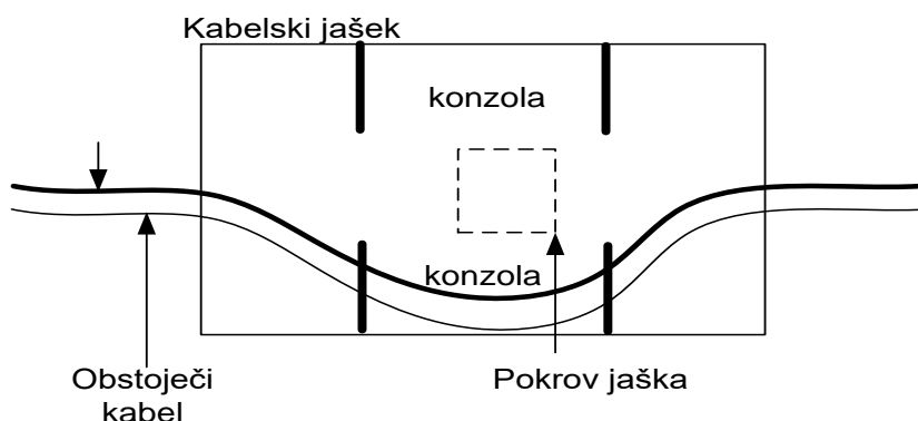
Slika 24: Pravilni prehod skozi jašek
