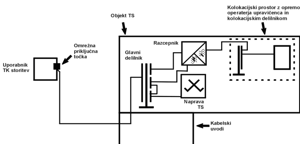
Slika 11: Sodiostop do bakrene krajevne zanke
