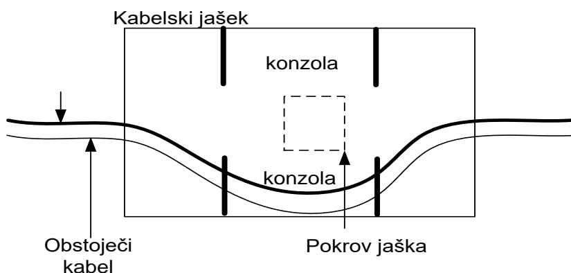
Slika 25: Pravilni prehod skozi jašek
