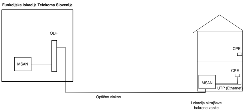
Slika 3: Topologija skrajšave zanke v dostopovnem bakrenem kabelskem omrežju – tip FTTP
