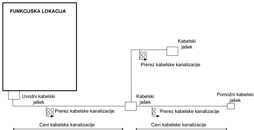
Slika 7: Kabelska kanalizacija
