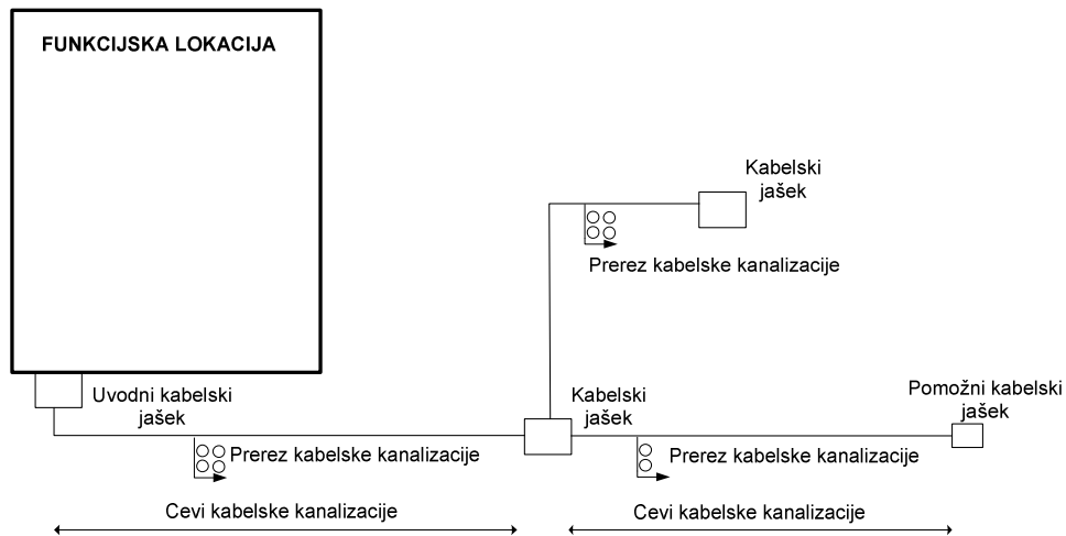
Slika 7: Kabelska kanalizacija
