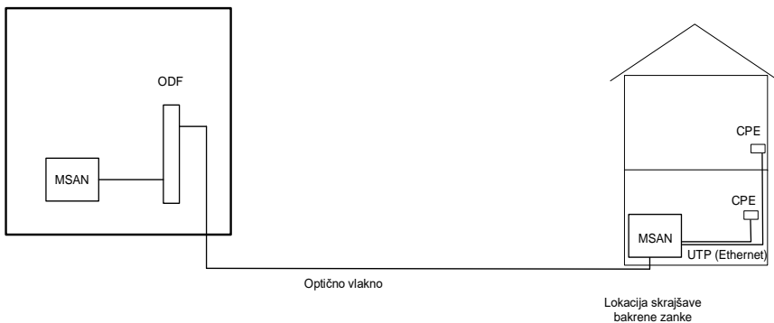
Slika 3: Topologija skrajšave zanke v dostopnem bakrenem kabelskem omrežju – tip FTTDp
