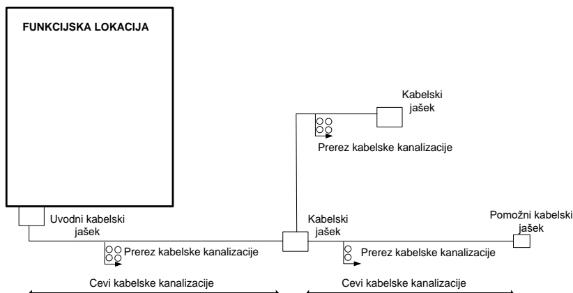
Slika 7: Kabelska kanalizacija
