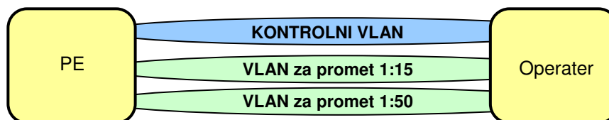
Slika 2: Logična konfiguracija povezave Telekom Slovenije - operater
