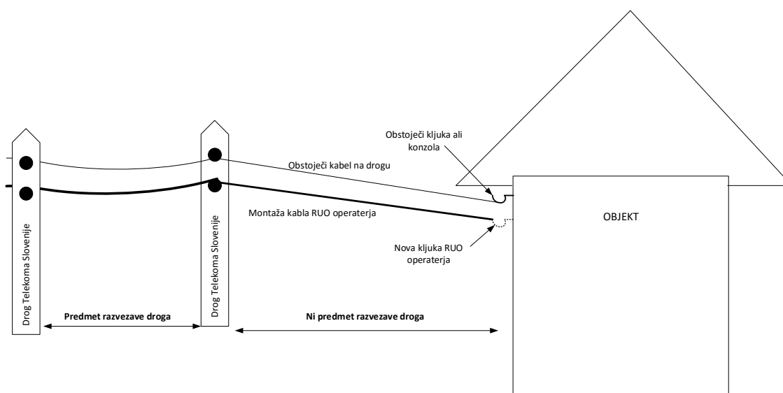
Slika 23: Razmejitvena točka med drogom in objektom
