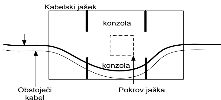
Slika 21: Pravilni prehod skozi jašek
