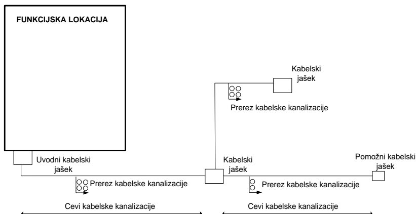
Slika 7: Kableska kanalizacija
