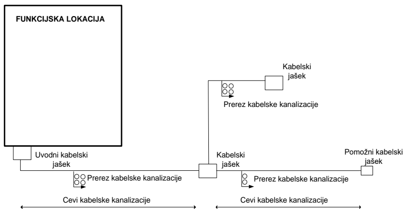
Slika 7: Kabelska kanalizacija
