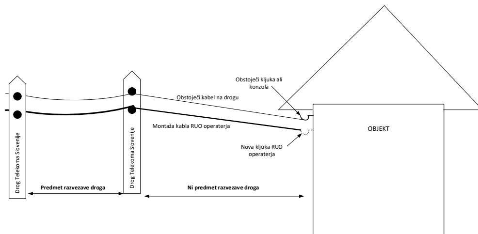
Slika 27: Razmejnitvena točka med drogom in objektom
