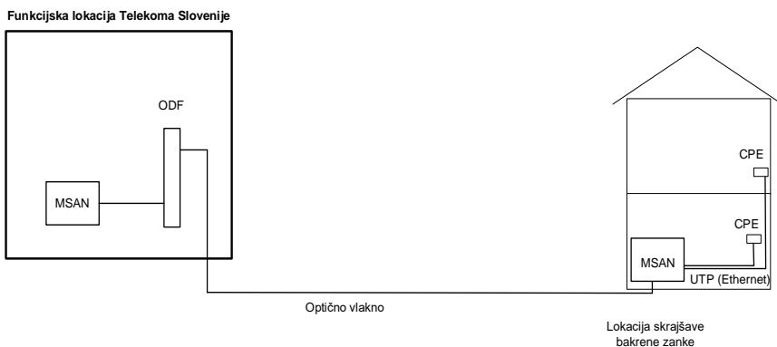
Slika 3: Topologija skrajšave zanke v dostopovnem bakrenem kabelskem omrežju – tip FTTdp
