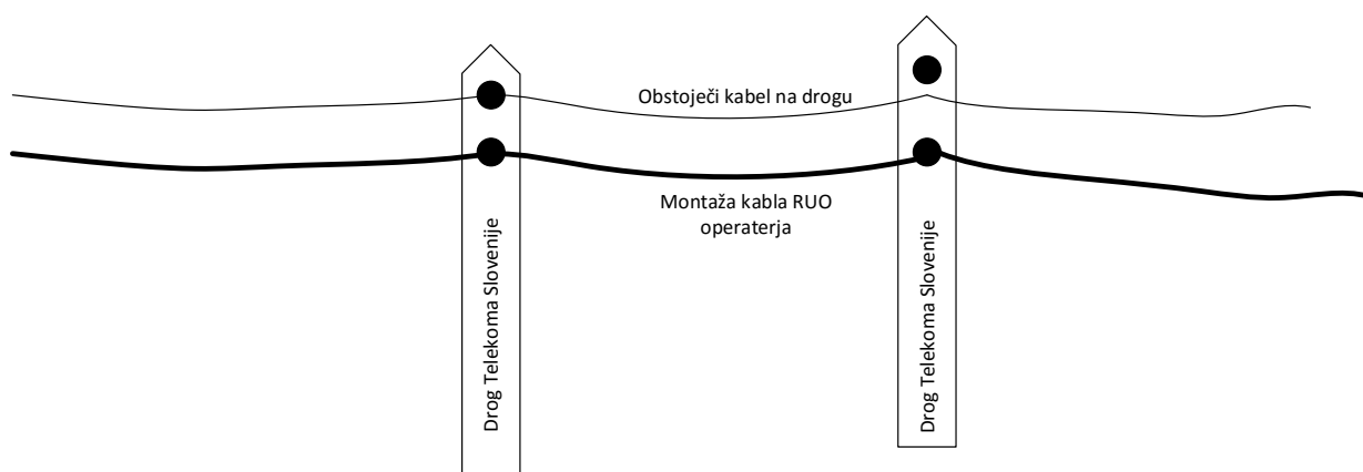
Slika 25: Pravilni prehod kabla na drogu
