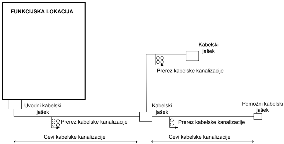
Slika 7: Kabelska kanalizacija
