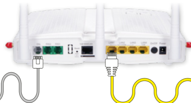
Slika 7: Povezava s sivim telefonskim kablom
