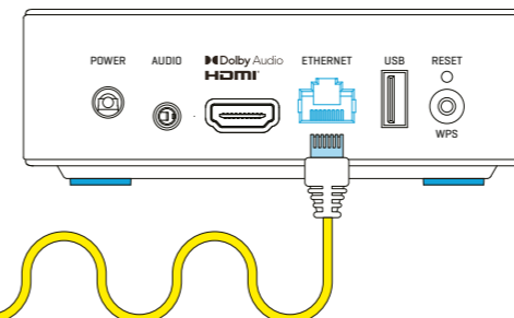
Slika 8: Povezava modema in NEO Smartboxa
